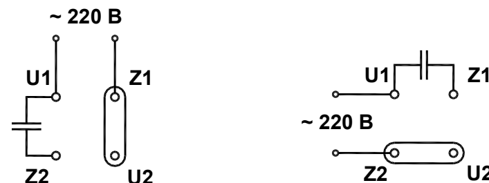
Схемы соединений на клеммной колодке двигателя
